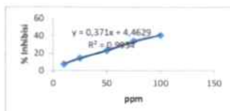
Gambar 1. Kurva Hasil Uji Antioksidan Ekstrak Air Daun Kelor
