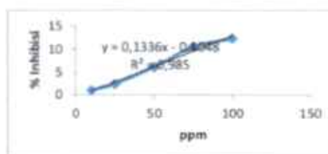
Gambar 2. Kurva Hasil Uji Antioksidan Ekstrak Air Buah Bit
